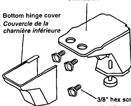
Bottom hinge Charnière inférieure
